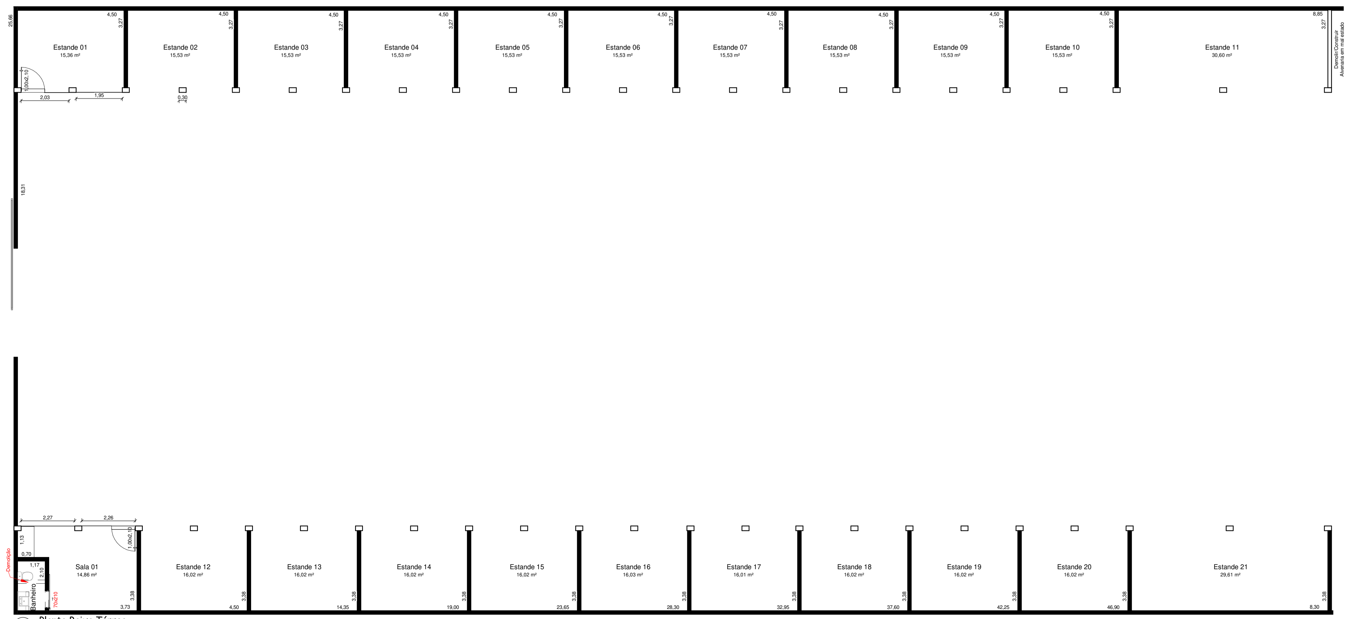
1 Planta Baixa Térreo 1 : 100
