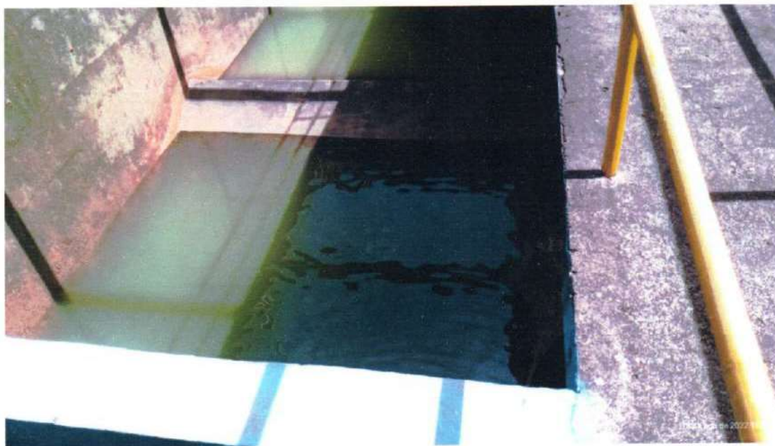
Figura 12; limpeza de decantador da eta principal.
