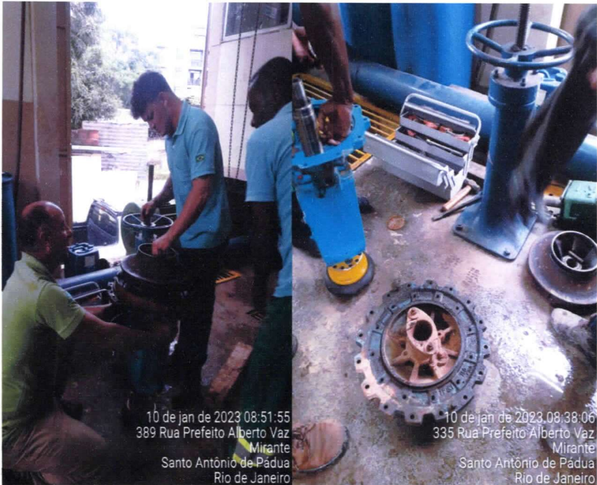
Figura 12 e 13 ; Manutenção preventiva da bomba e motor da captação principal no município.
