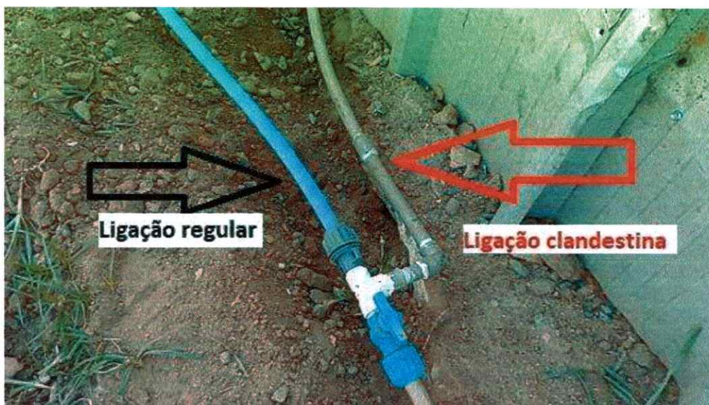
Figura 5: Ligação clandestina realizada em ramal de abastecimento de hidrômetro
