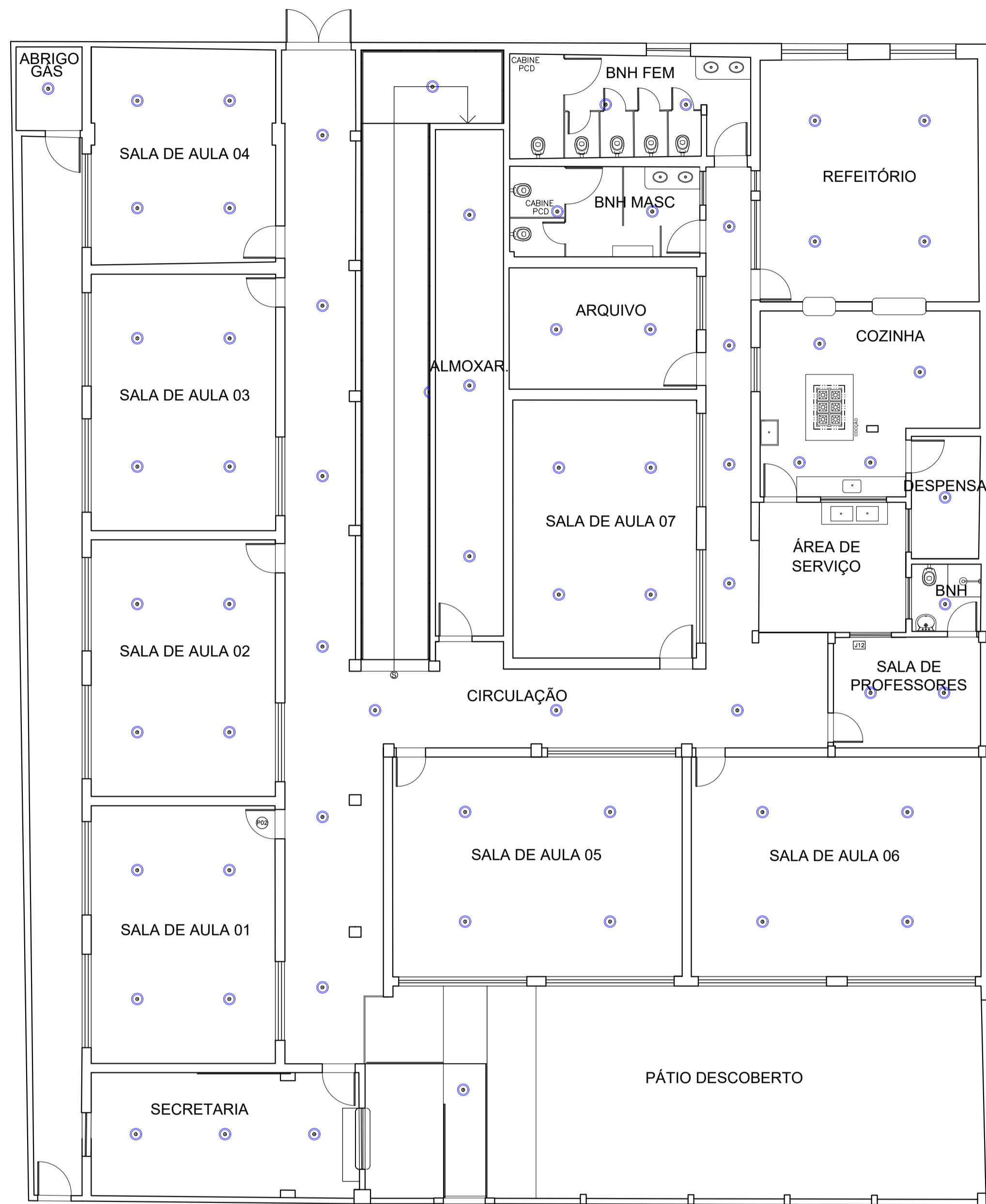
14 PLANTA DE PONTOS DE ILUMINAÇÃO - PAV. TÉRREO ESCALA 1:100
