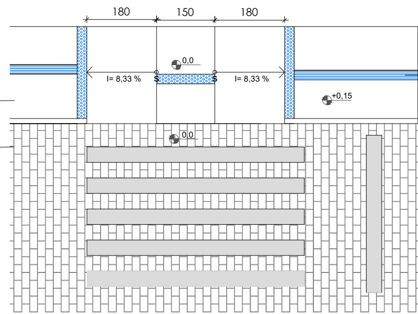
DETALHE - RAMPA DE ACESSO
