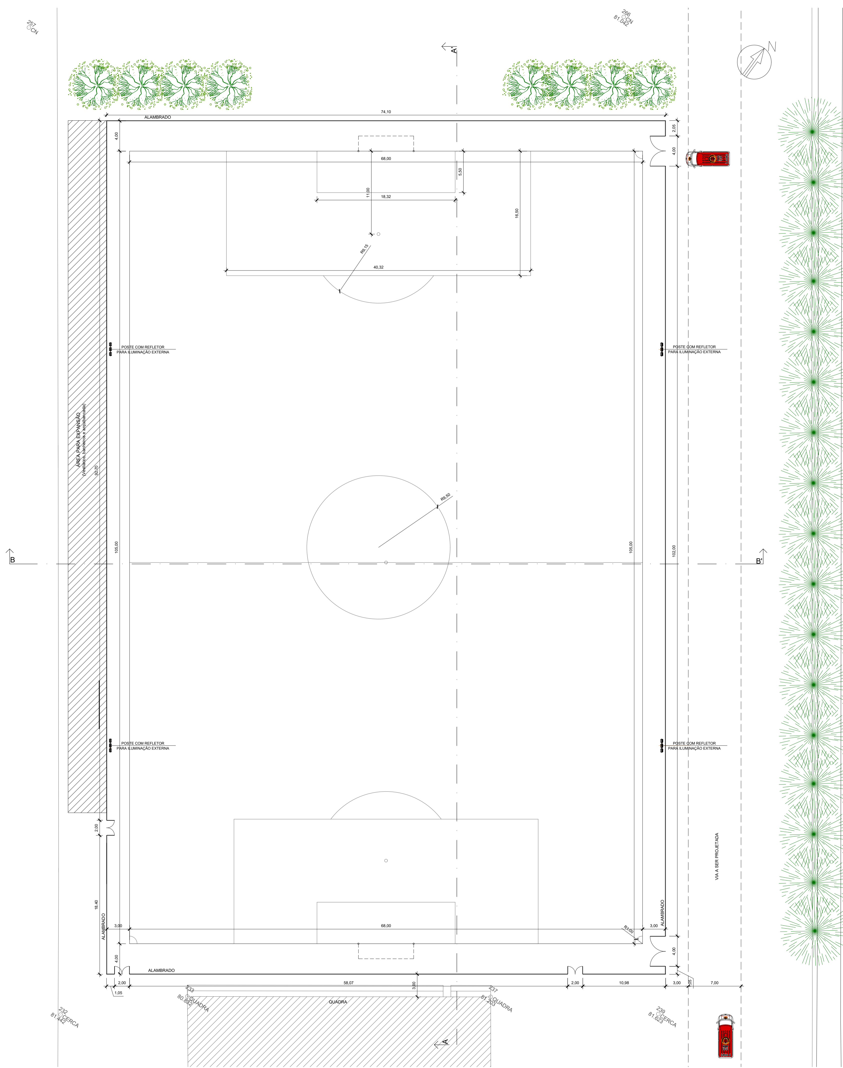
PLANTA BAIXA - CAMPO DE FUTEBOL Esc. 1/250
