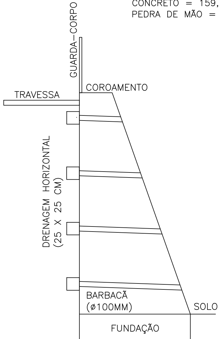
CORTE - DRENAGEM
