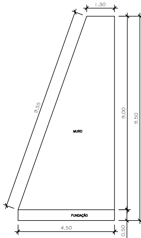
VISTA LATERAL
